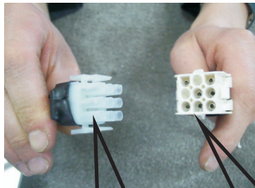
Kábel odsávača
