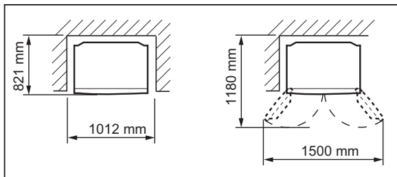
Celkový prostor potřebný při provozu
